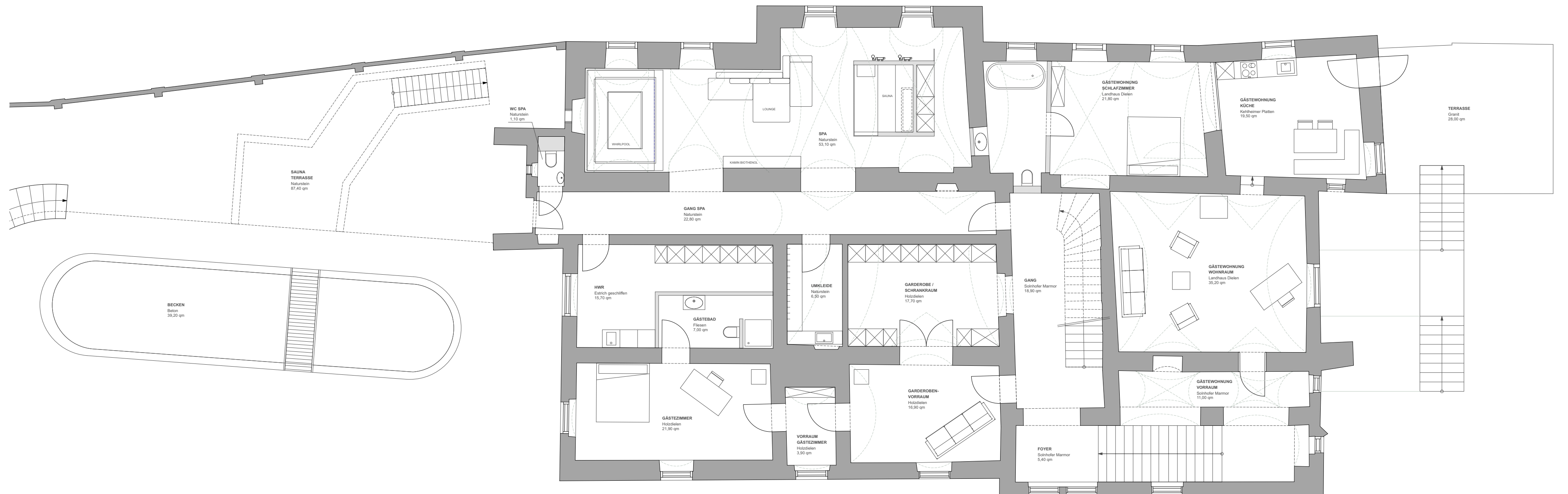
ERDGESCHOSS M 1:100
