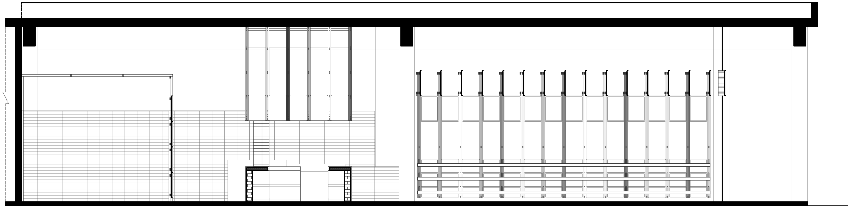
MI PAN / CORTE B - B'
