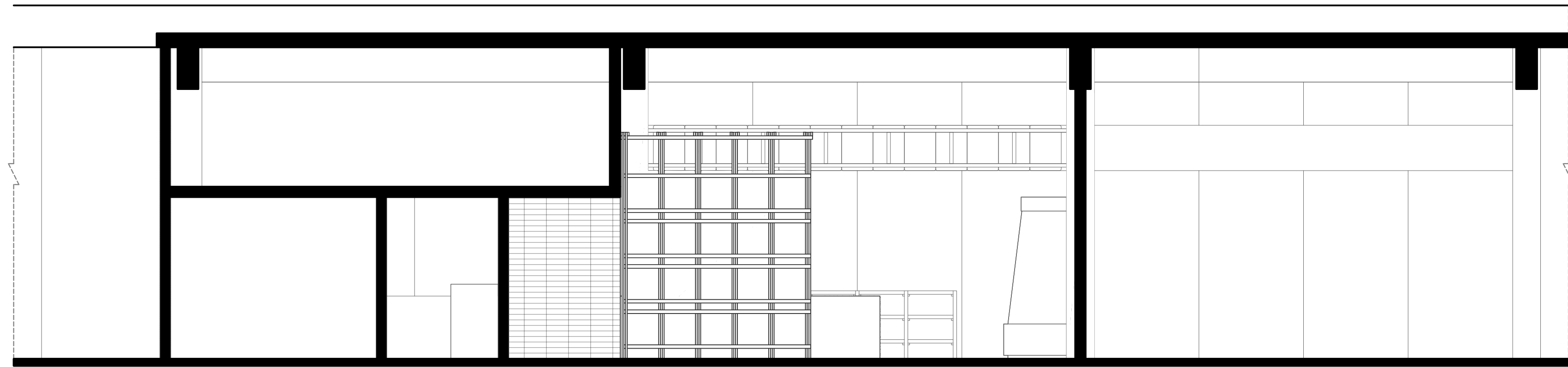
MI PAN / CORTE J - J'
