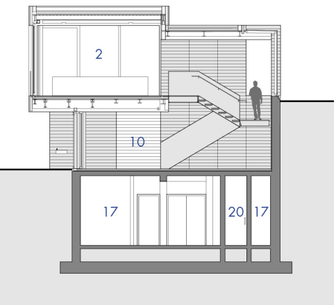
Coupe transversale Cross-section
