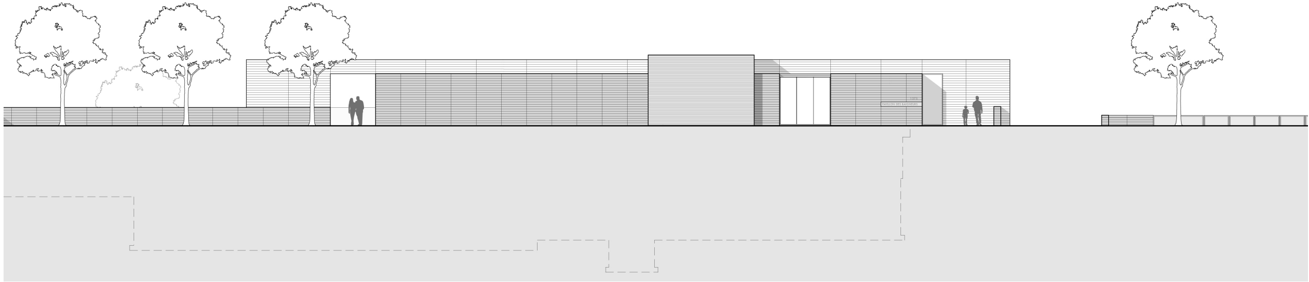
Élévation ouest West Elevation
