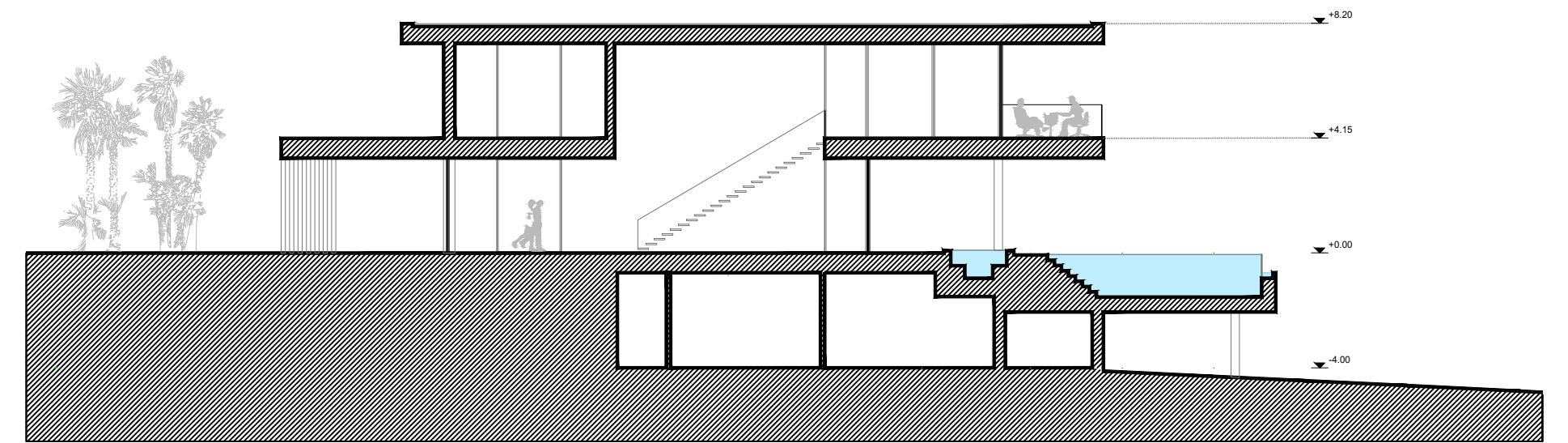
SECTION A-A
