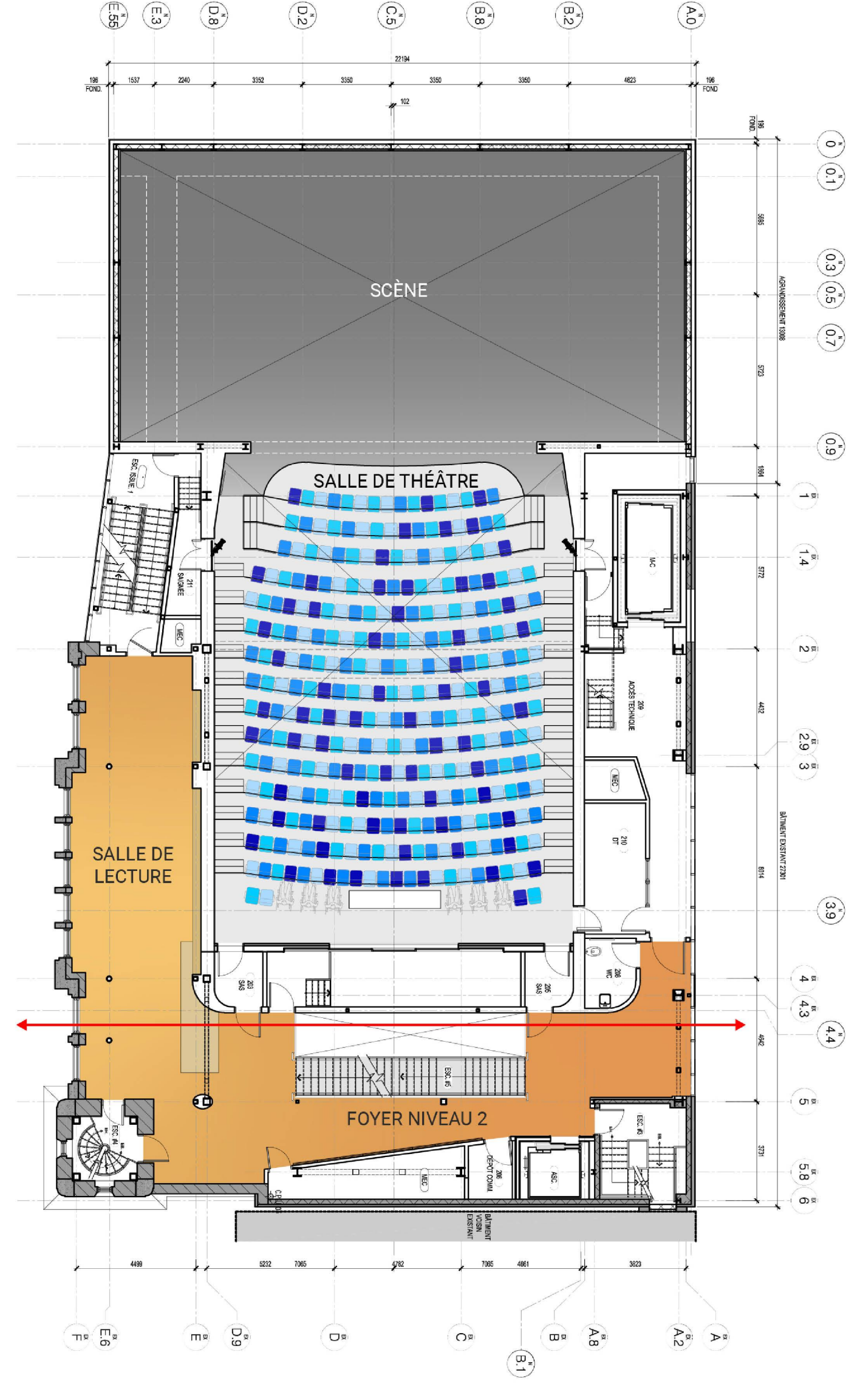
NIVEAU 2
