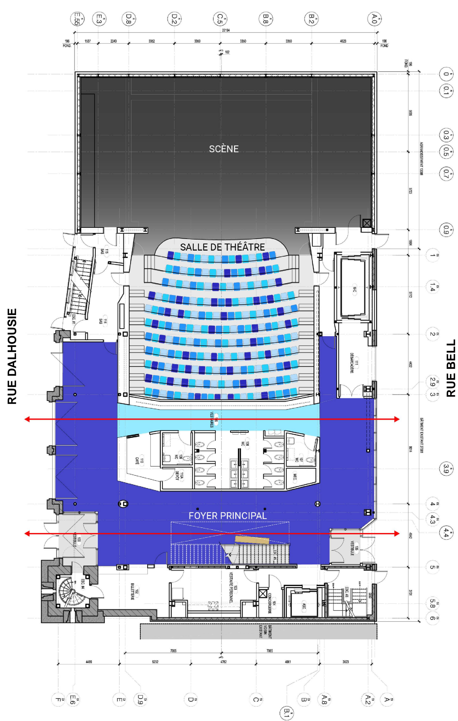
REZ-DE-CHAUSSÉE
