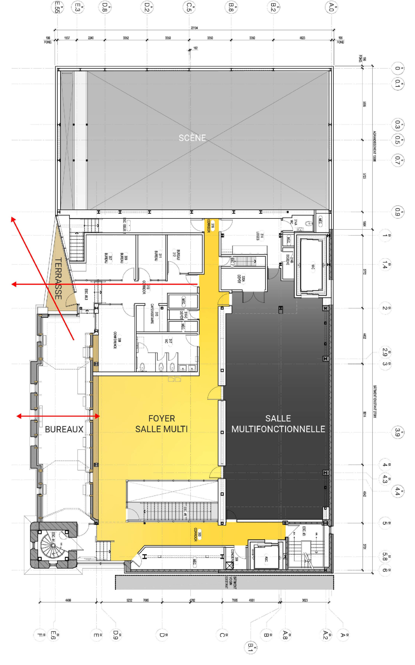
NIVEAU 3
