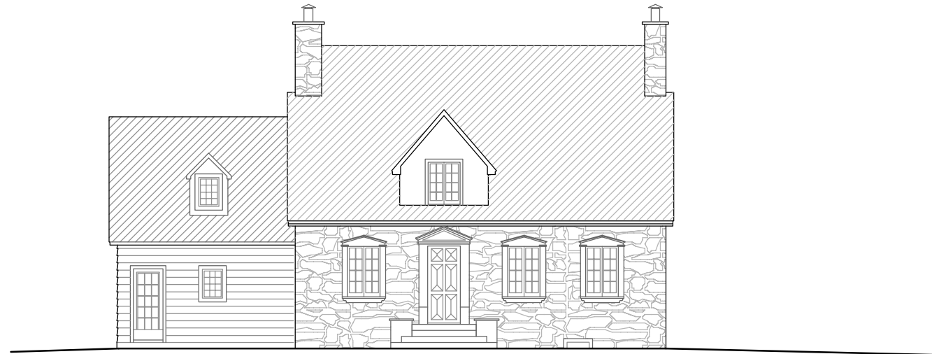
ÉLEVATION OUEST - EXISTANT 0' 5' 20'
