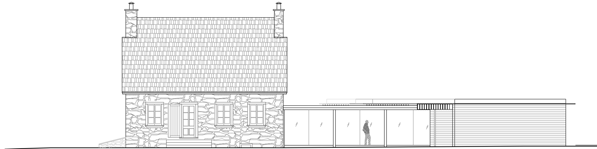
ÉLEVATION OUEST - AGRANDISSEMENT
