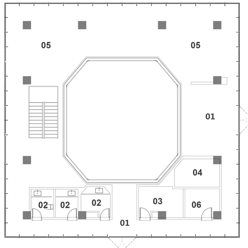
一层平面图 1F Layout Plan
