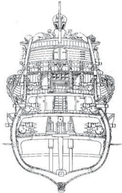
Schnitt Spant 6
