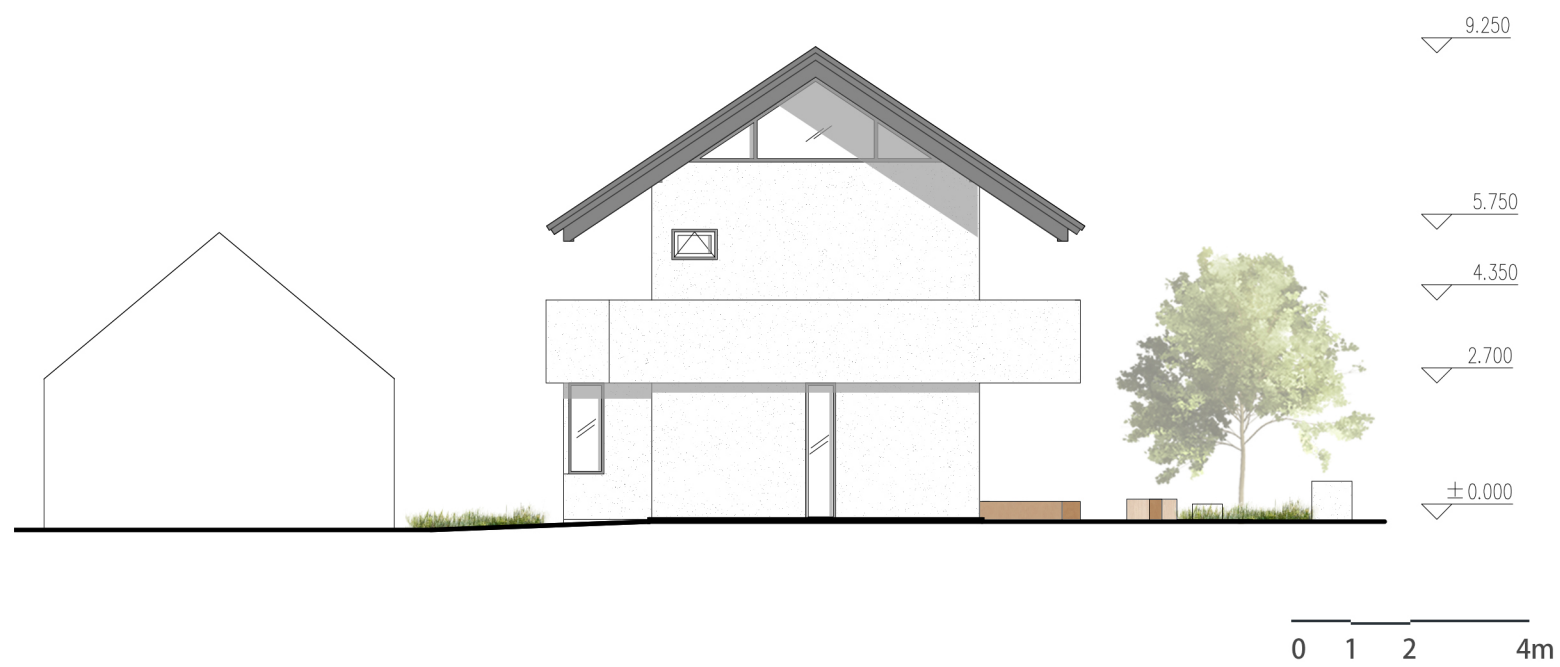
西立面 West Elevation
