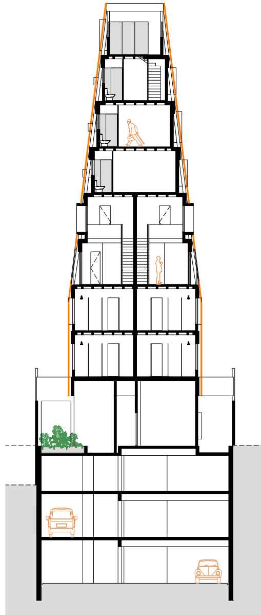
CORTE BB
