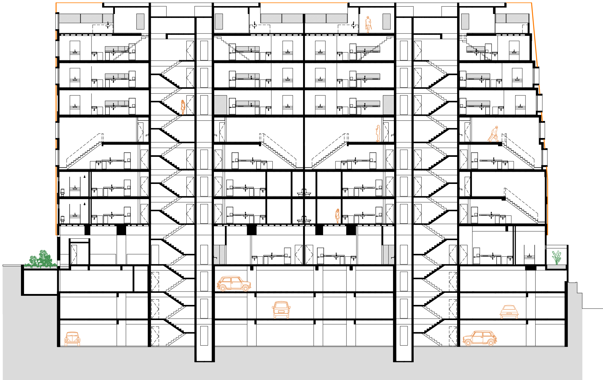
CORTE AA
