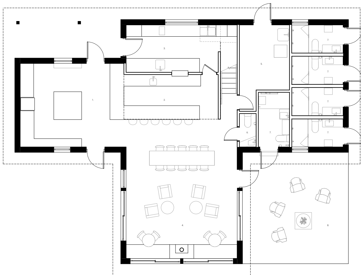
PLAN REZ-DE-CHAUSSEE
