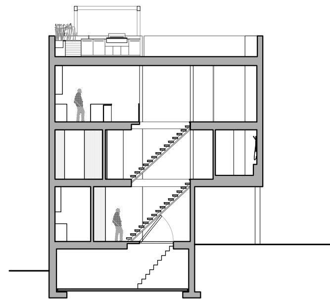
COUPE 2 0' 5' 20'
