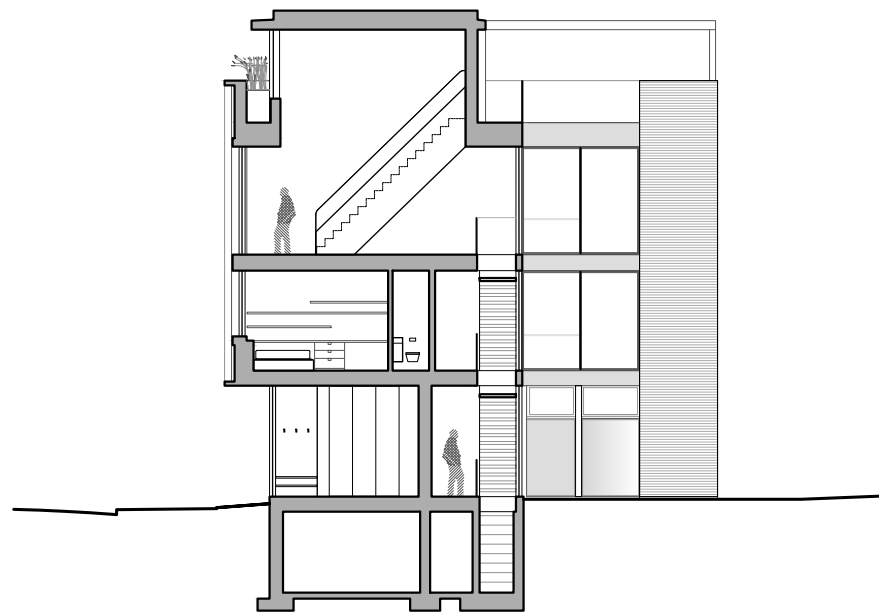
COUPE A 0' 5' 20'
