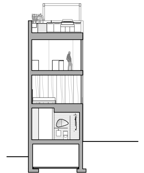
COUPE 3 0' 5' 20'
