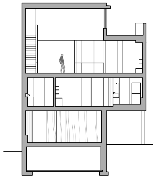
COUPE 1 0' 5' 20'
