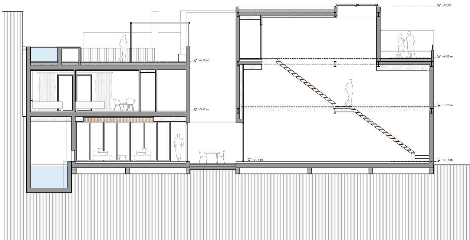
SECCIÓN LONGITUDINAL
