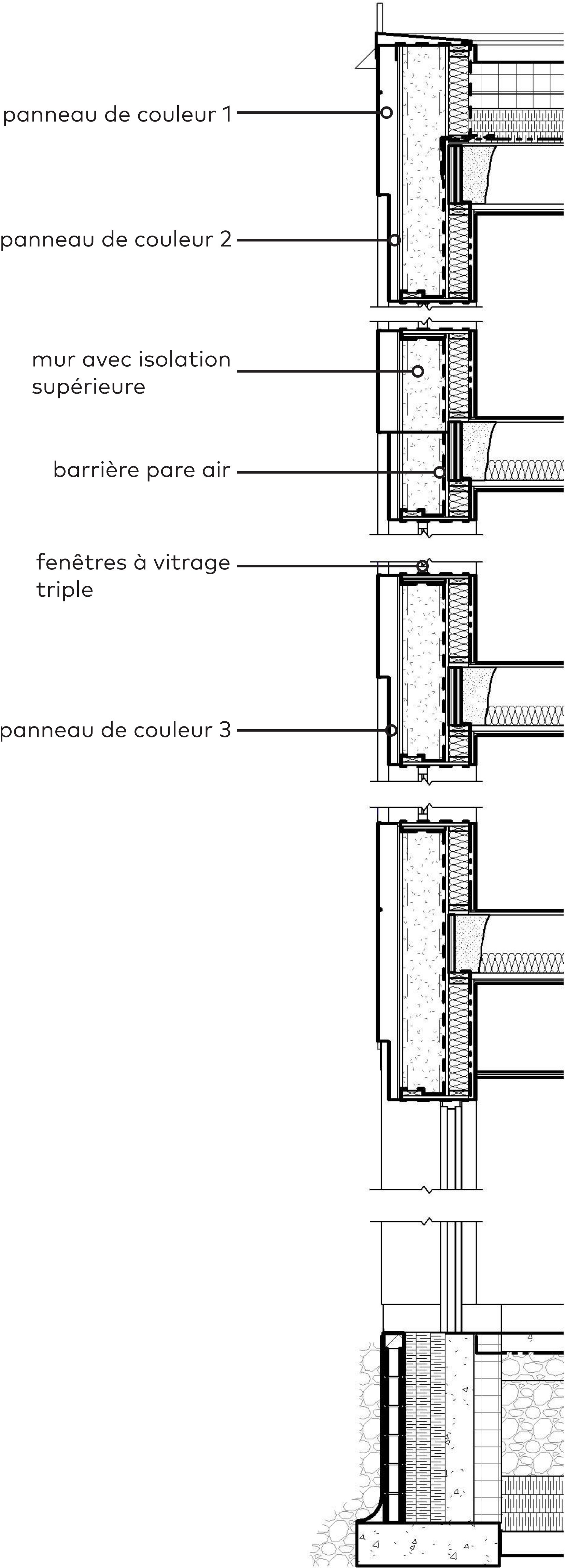
Coupe de mur (1:50)
