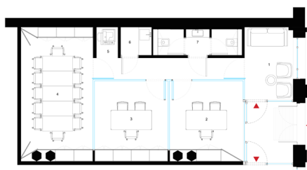
Plan 1 | 2 | 3 | 4 | 5 | 6 | 7 accueil | bureau | bureau | salle de réunion | photocopieur | cuisine | wc
