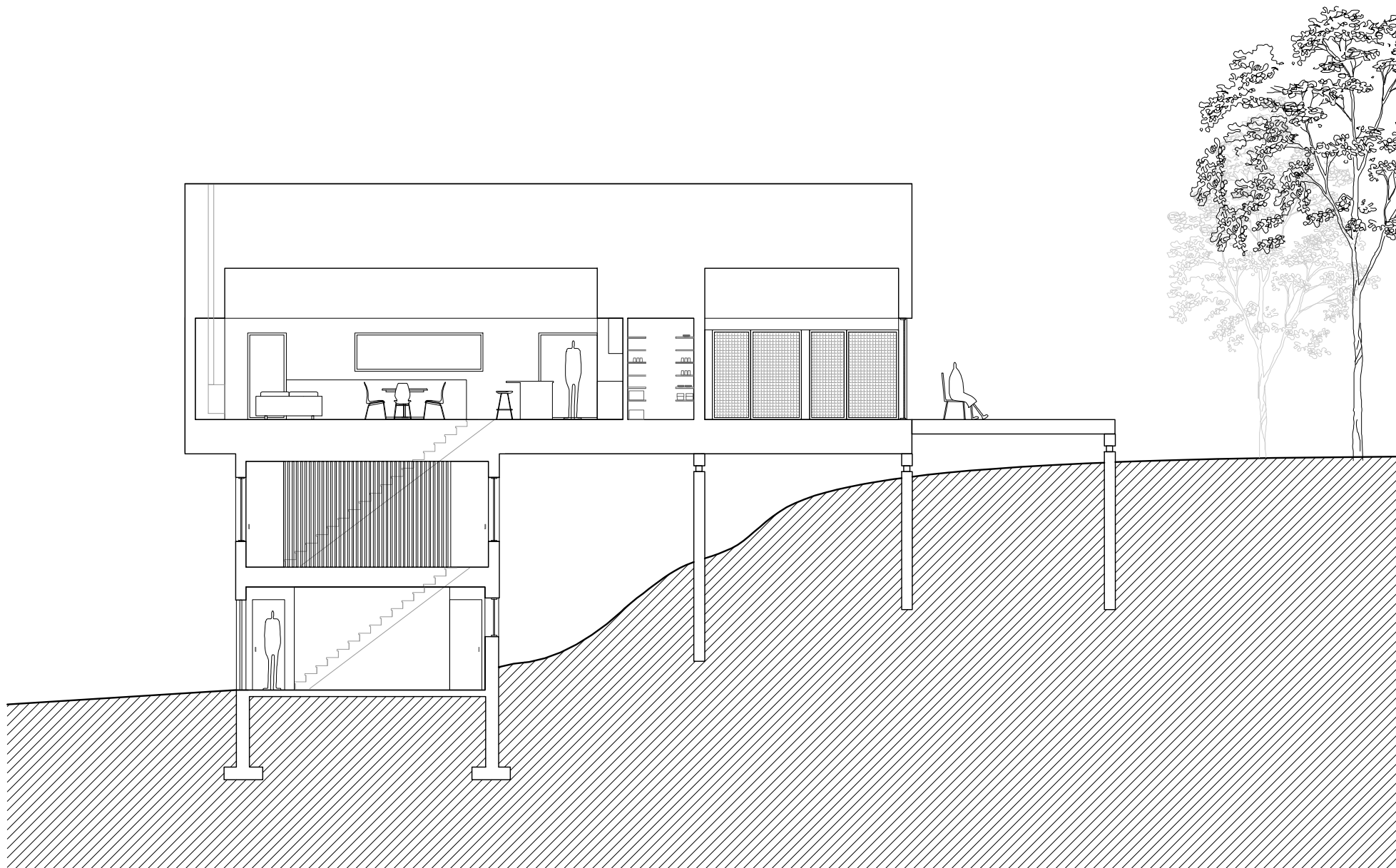
Coupe transversale
