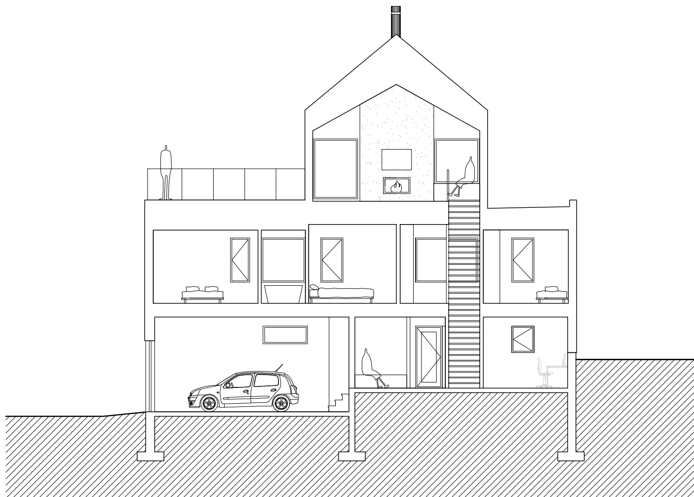
Coupe longitudinale 0 1 2 5 10 20 (pi)
