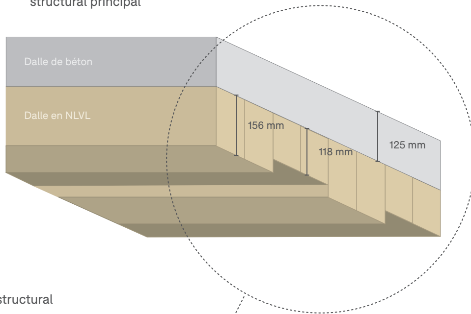
B Détail du système structural principal
