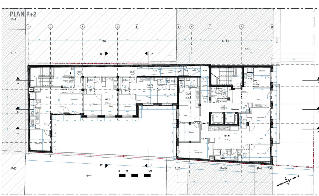
Plan R+2
